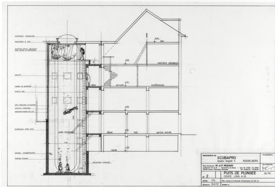
8. Marcel et Paul Mignot, projet de puits de plongée pour la société Scubapro, 1972 ©AAM, Bruxelles Marcel & Paul Mignot, ontwerp voor een duikput voor de onderneming Scubapro, 1972 ©AAM, Brussel
